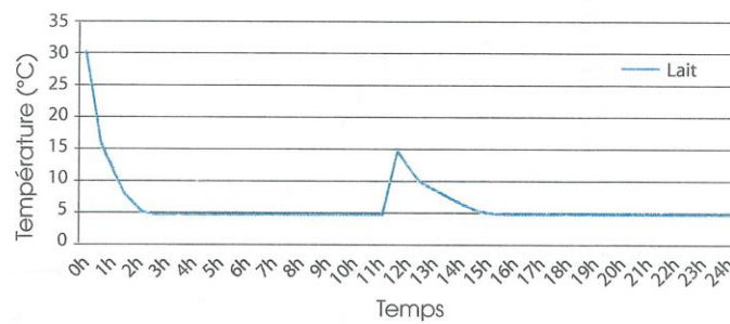
Courbes des Températures pour 2 traites
