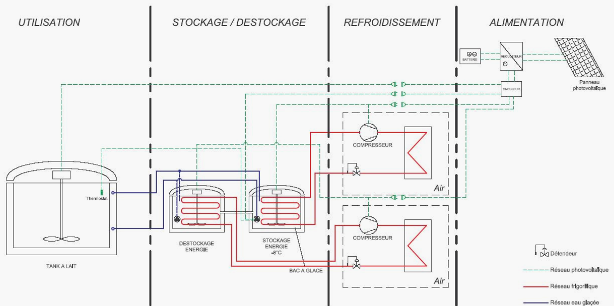
Système prêt à brancher - Circuit frigorifique simple*
